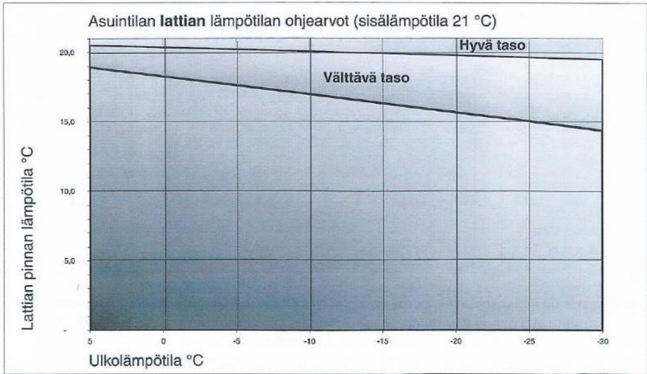
Kuva 2. Asuintilan lattian lämpötilojen tason arviointi eri ulkolämpötiloissa kun sisälämpötila on 21 °C.
