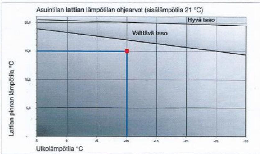
Kuva 2. Asuintilan lattian lämpötilojen tason arviointi eri ulkolämpötiloissa kun sisälämpötila on 21 °C.
